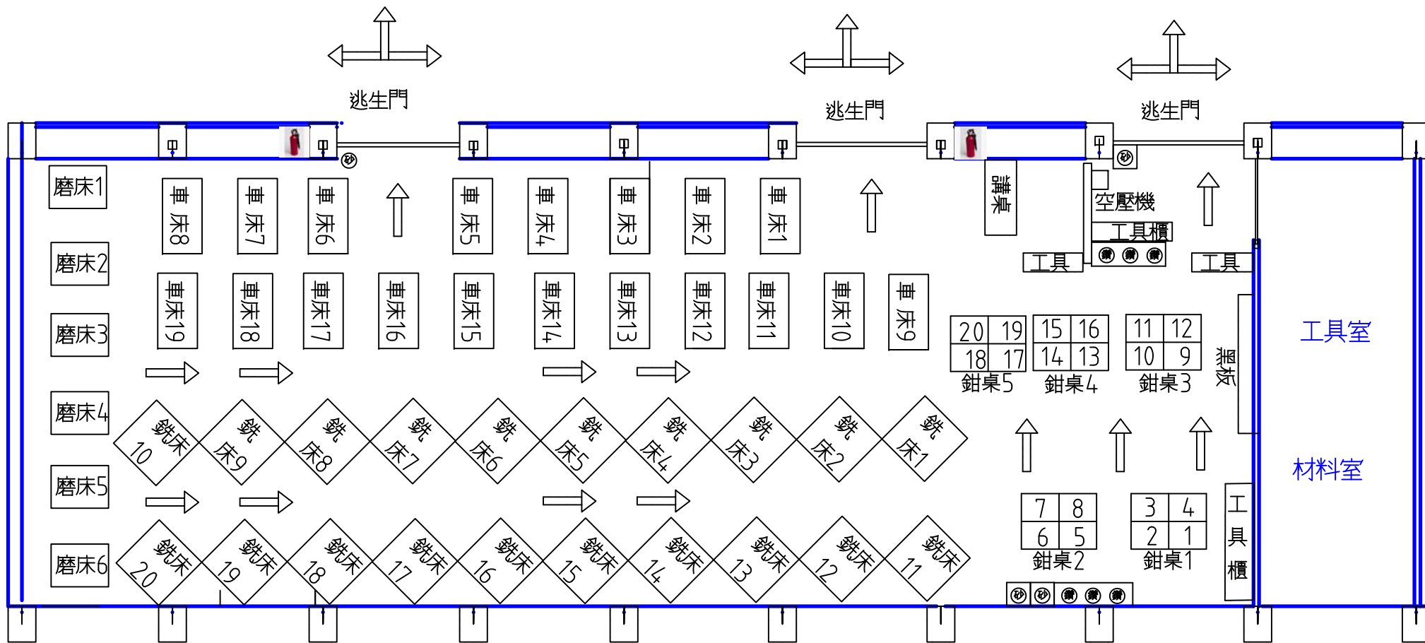
機械科第二工場工作崗位位置圖暨逃生平面路線圖
