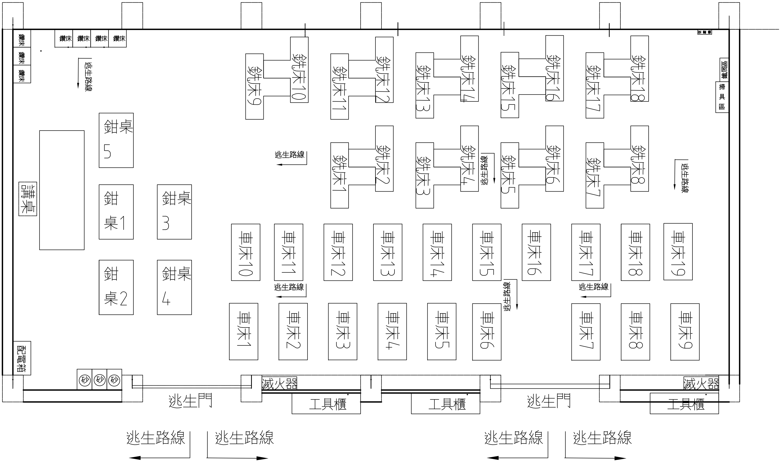
第一工場車床丙級工作崗位位置圖
